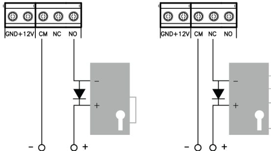
Рис.7. Подключение замков
